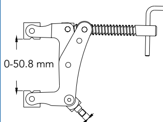
EXT M6
