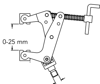
EXT M6
