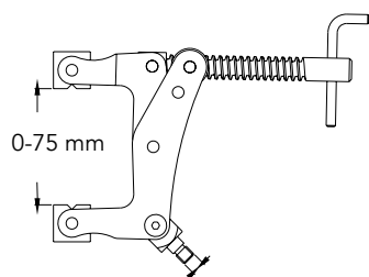
EXT M8
