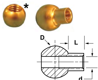
foro filettato diritto
